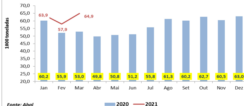
Indústria de Alumínio Produção mensal de alumínio primário
